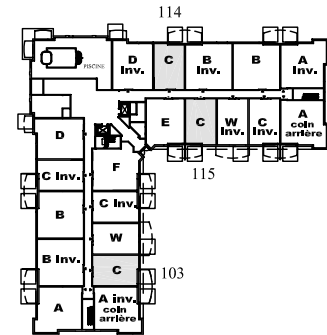
REZ-DE-CHAUSSÉE
