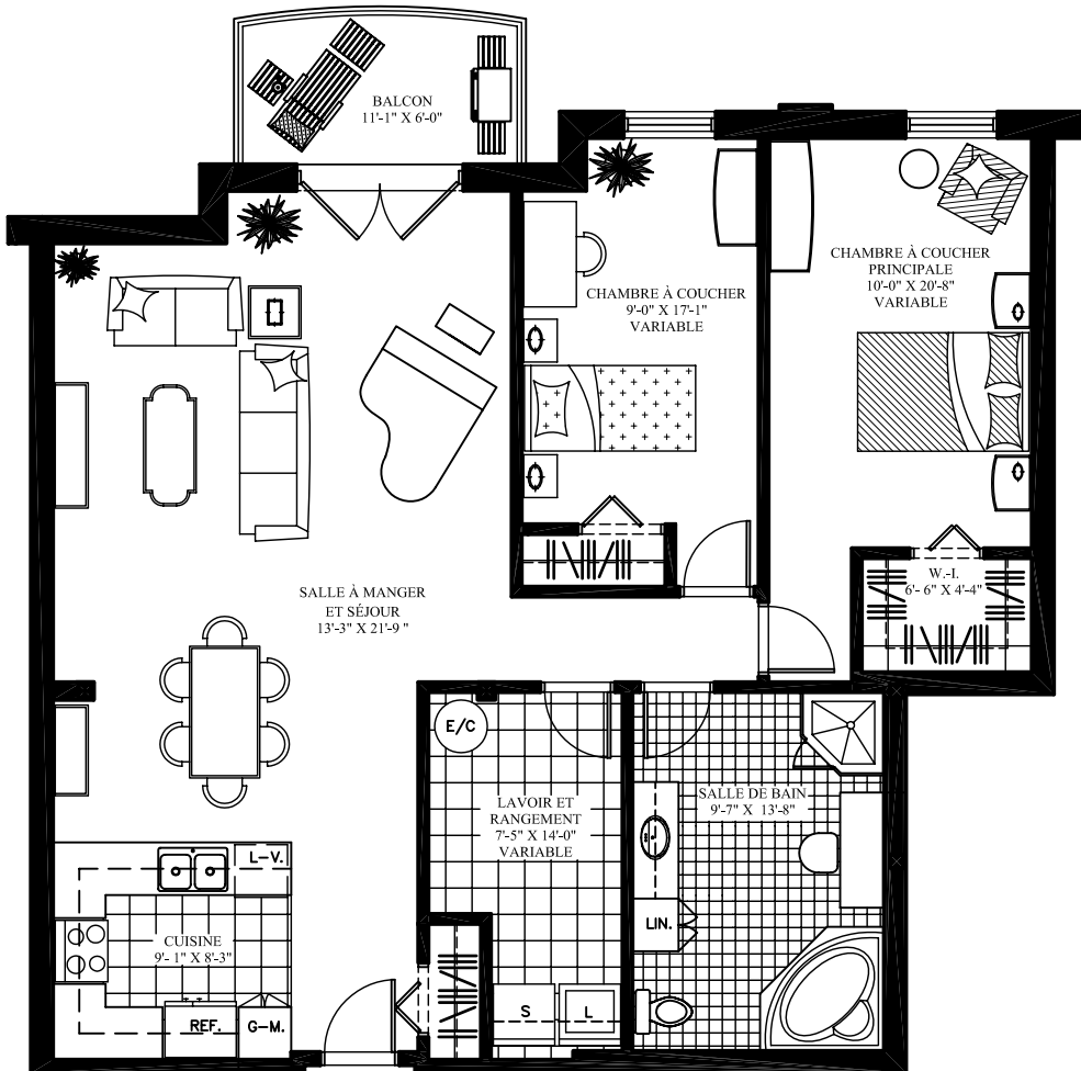
3e-4e-5e ÉTAGE
